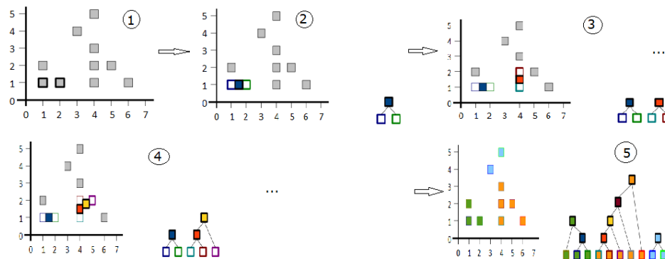
FIGURE 2.2 – Exemple en dimension 2 d'une classification hiérarchique ascendante
